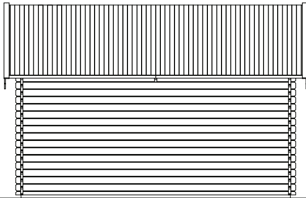
achteraanzicht / rear view
