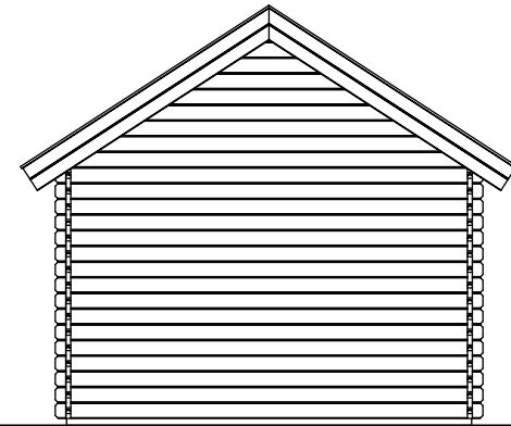
(L) zijaanzicht / side view
